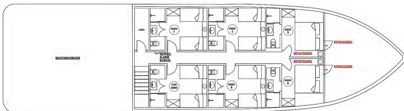
UNTERDECK
