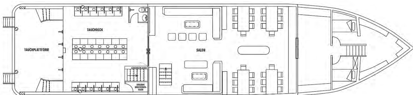
HAUPTDECK
